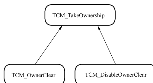
图 4 Owner 管理命令依赖关系
