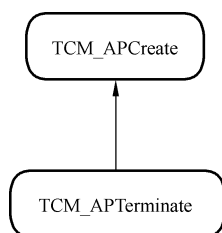
图 15 授权协议命令依赖关系
