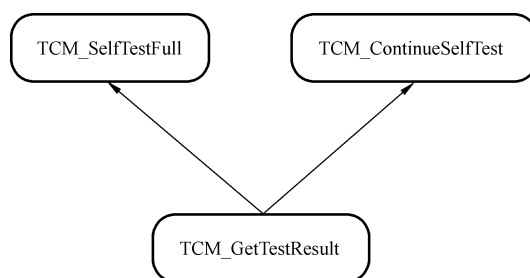
图 3 自检命令依赖关系
