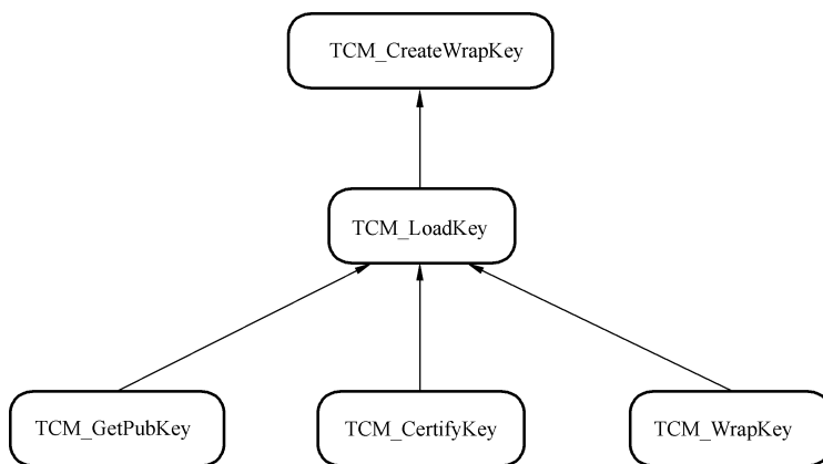
图 10 密钥管理命令依赖关系
