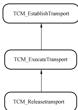
图 14 传输会话命令依赖关系
