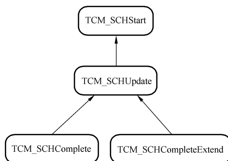
图 13 密码服务命令依赖关系
