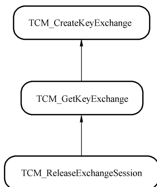
图 11 密钥协商命令依赖关系
