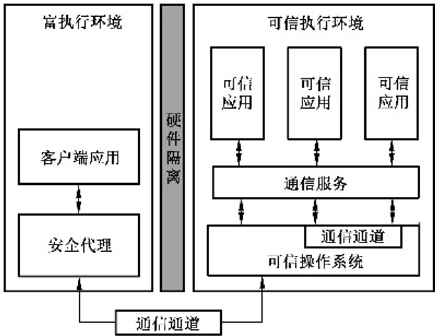
图 5 可信应用通信框架
