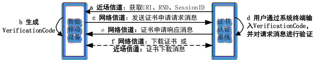
图 2 证书申请协议流程图
