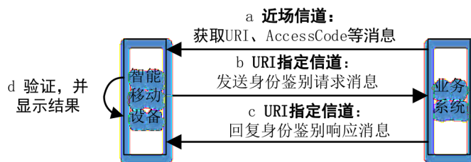
图 5 用于身份鉴别的数字签名验证流程图
