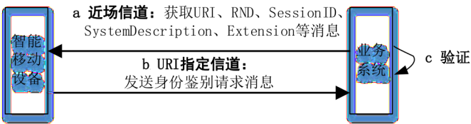
图 3 用于身份鉴别的数字签名协议流程图
