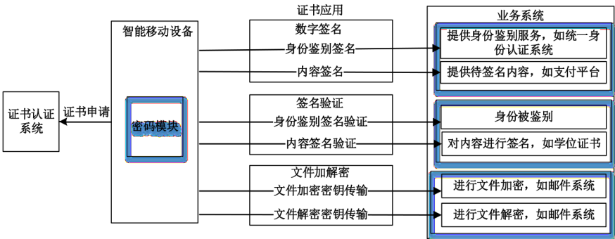
图 1 基于多信道的证书申请和应用协议框架图
