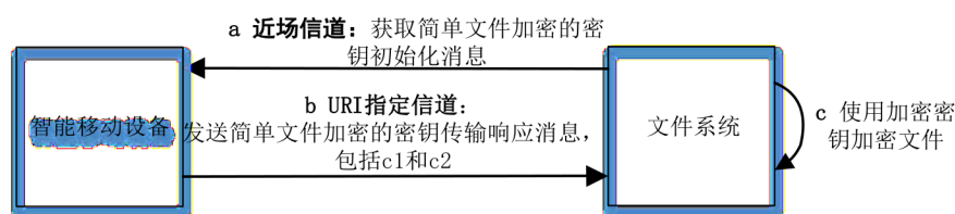
图 7 文件加密密钥传输协议流程图
