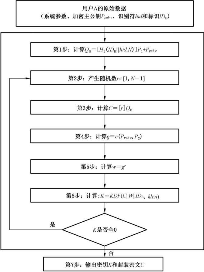
图 4 密钥封装算法流程
