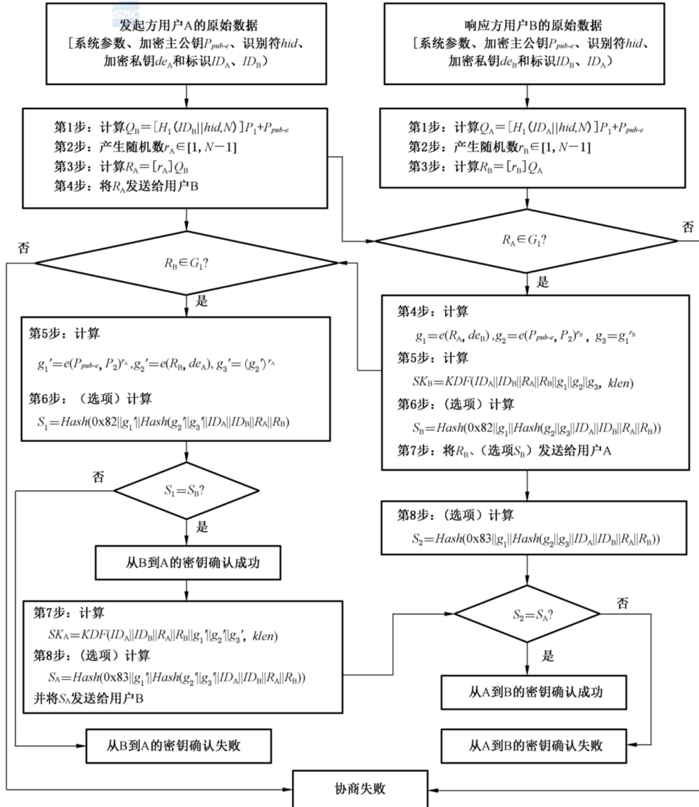
图 3 密钥交换协议流程
