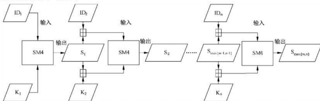
图 2 SM4 运算过程图
