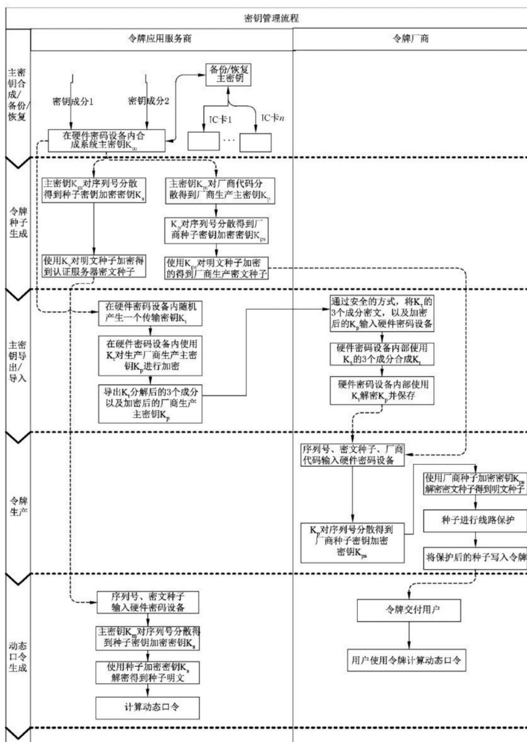
图 4 对称算法密钥管理示例流程图
