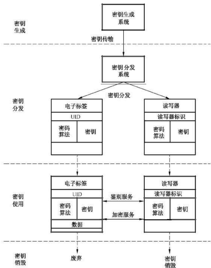
图 2 射频识别系统对称密钥管理模型
