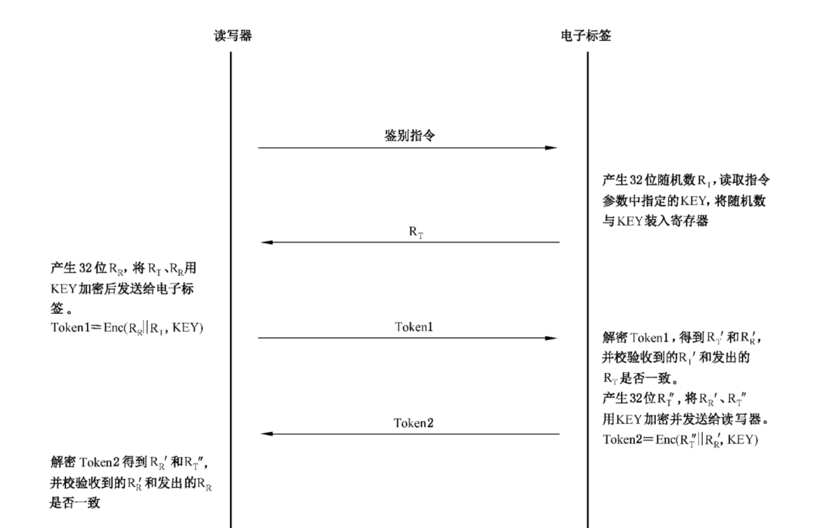
图 C.1 基于 SM7 对称密码算法的双向身份鉴别
