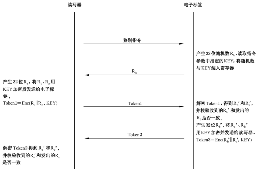
图 A.3 鉴别流程
