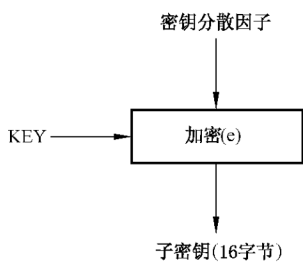
图 A.5 密钥分散计算方法
