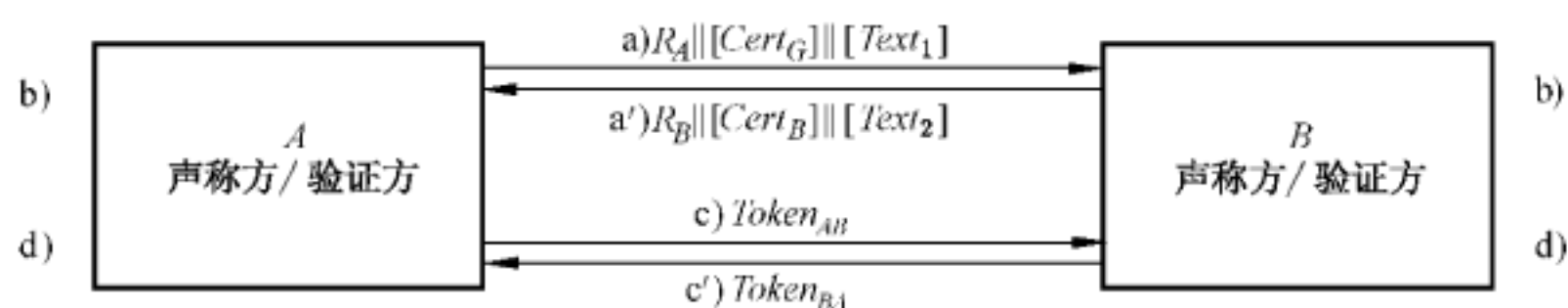
图9 两次传递并行的单向匿名双向鉴别
