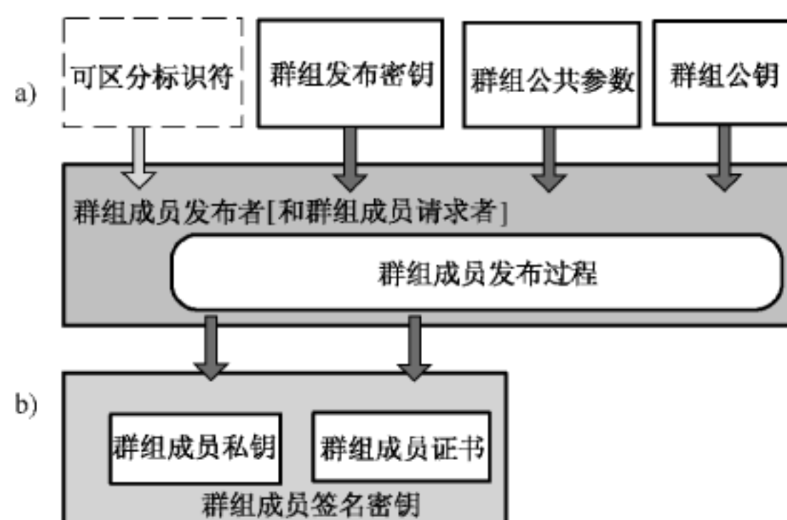
图 1 群组成员的发布过程
