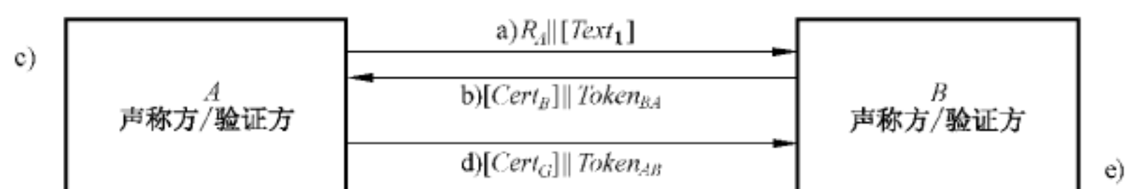
图 8 三次传递单向匿名双向鉴别
