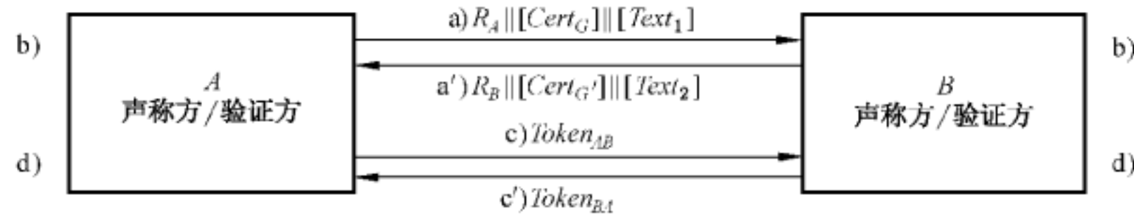
图 6 两次传递并行的双向匿名鉴别
