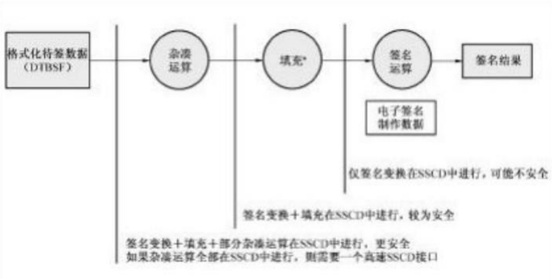
图 5 签名过程及在 SCA 和 SSCD 之间可能的工作分工
