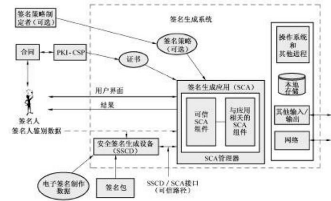
图 1 签名生成的功能模型
