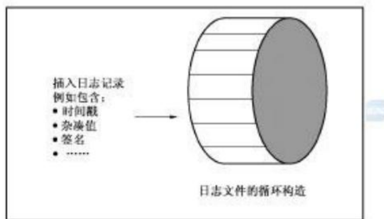
图 C.1 签名的日志
