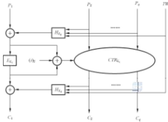
图 13 带泛杂凑函数的计数器工作模式加密算法
