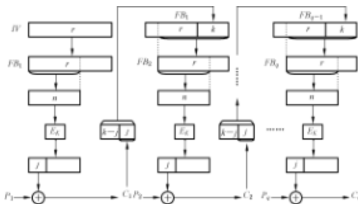
图 5 密文反馈工作模式加密算法
