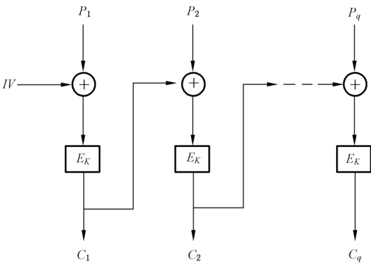
图 3 密文分组链接工作模式加密算法
