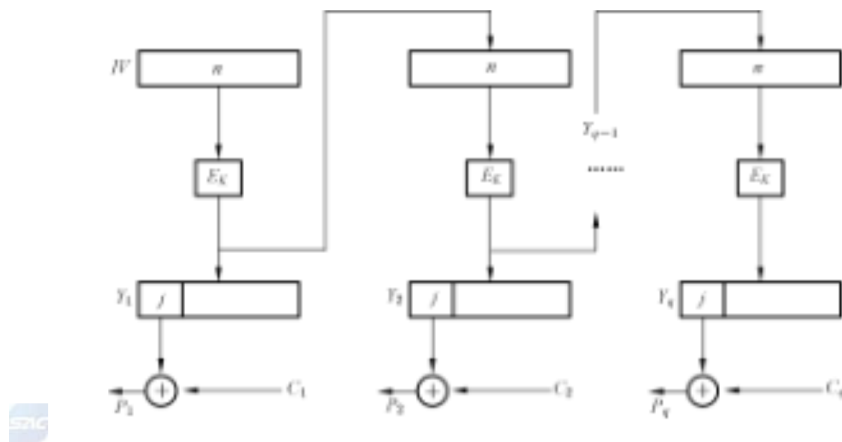
图 8 输出反馈工作模式解密算法
