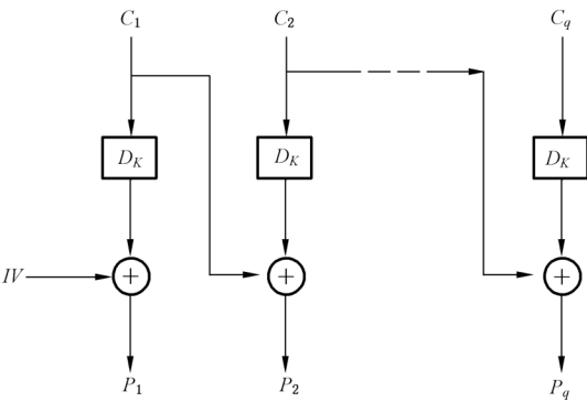
图 4 密文分组链接工作模式解密算法
