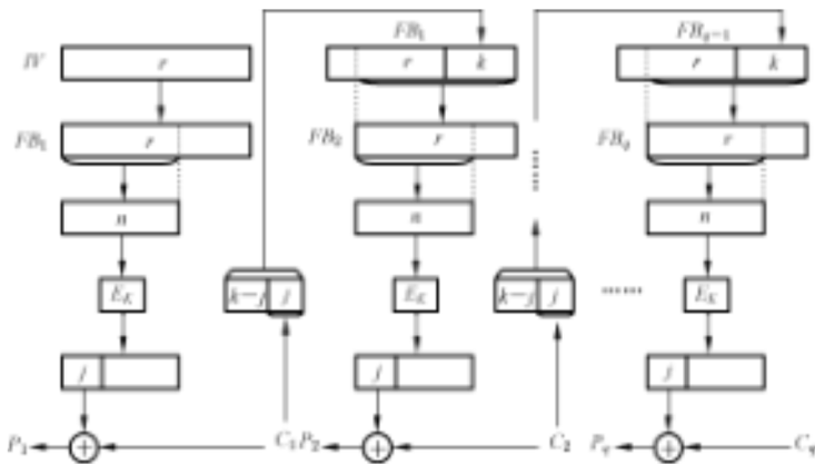
图 6 密文反馈工作模式解密算法
