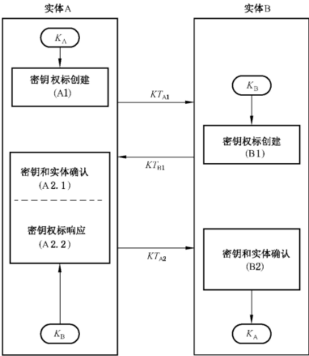
图 15 密钥传递机制 6
