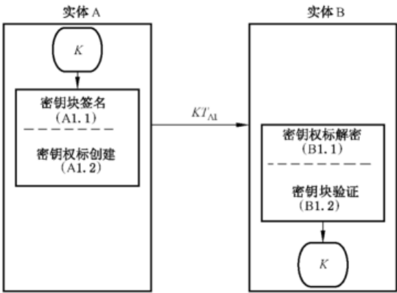
图 12 密钥传递机制 3
