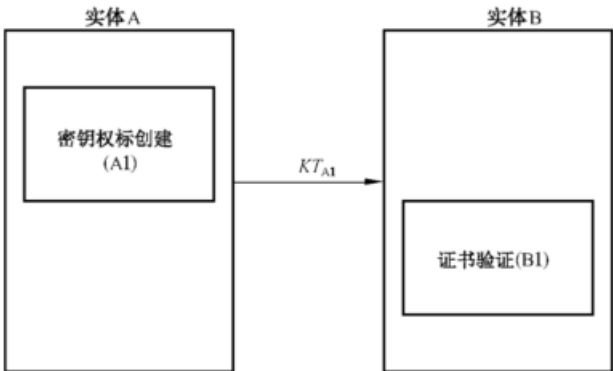
图 18 公钥传递机制 3
