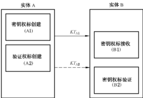
图 17 公钥传递机制 2
