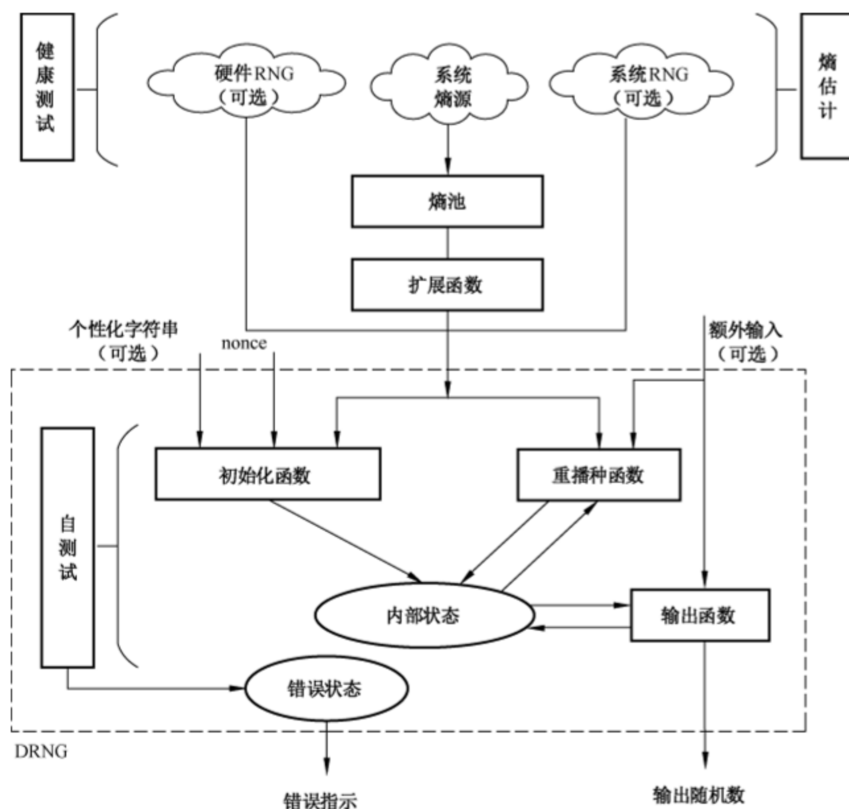
图 1 软件随机数发生器的基本模型
