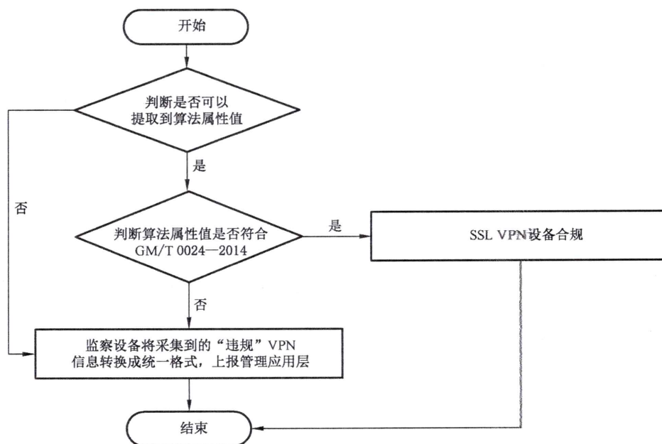
图 5 基于 SSL VPN 协议的检测流程图
