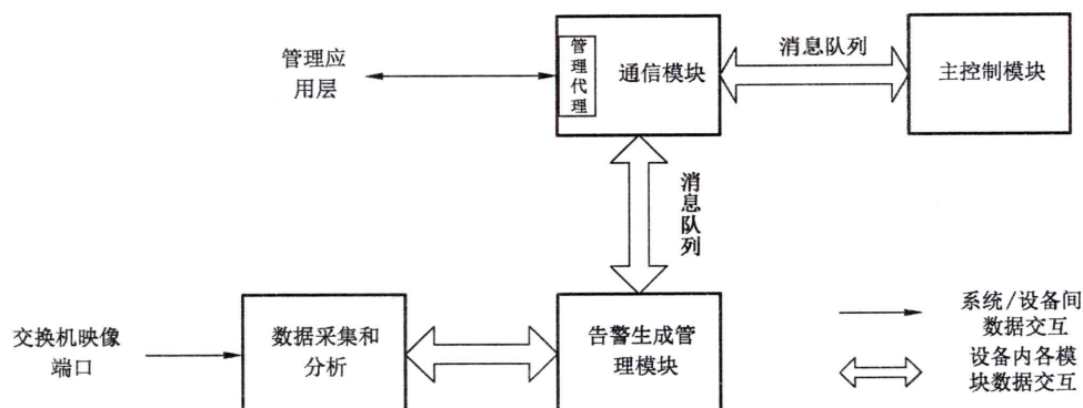
图 2 VPN 设备的监察设备示意图
