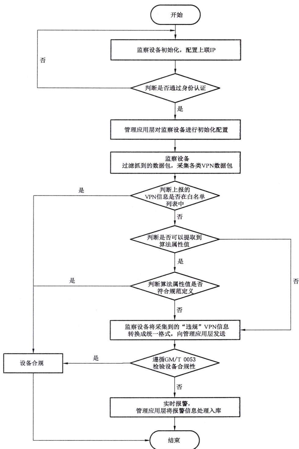
图3 监察管理系统工作流程图
