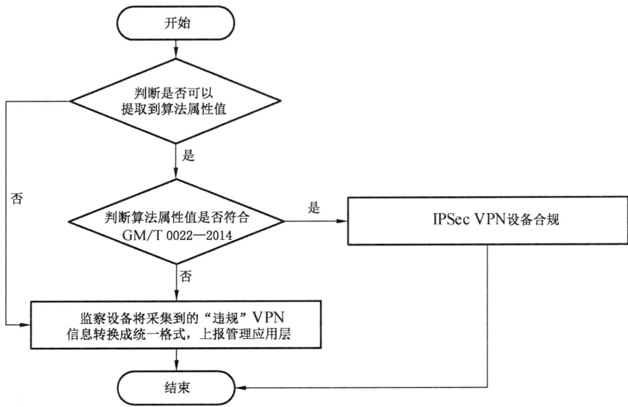
图 4 基于 IPSec VPN 协议的检测流程图
