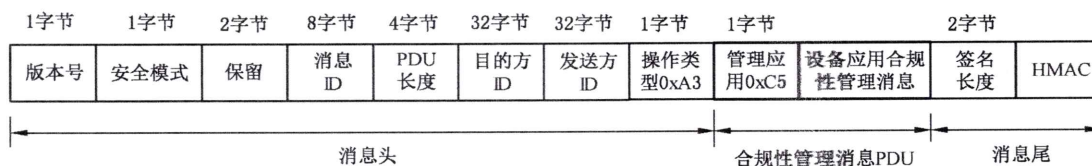
图 6 监察管理消息格式
