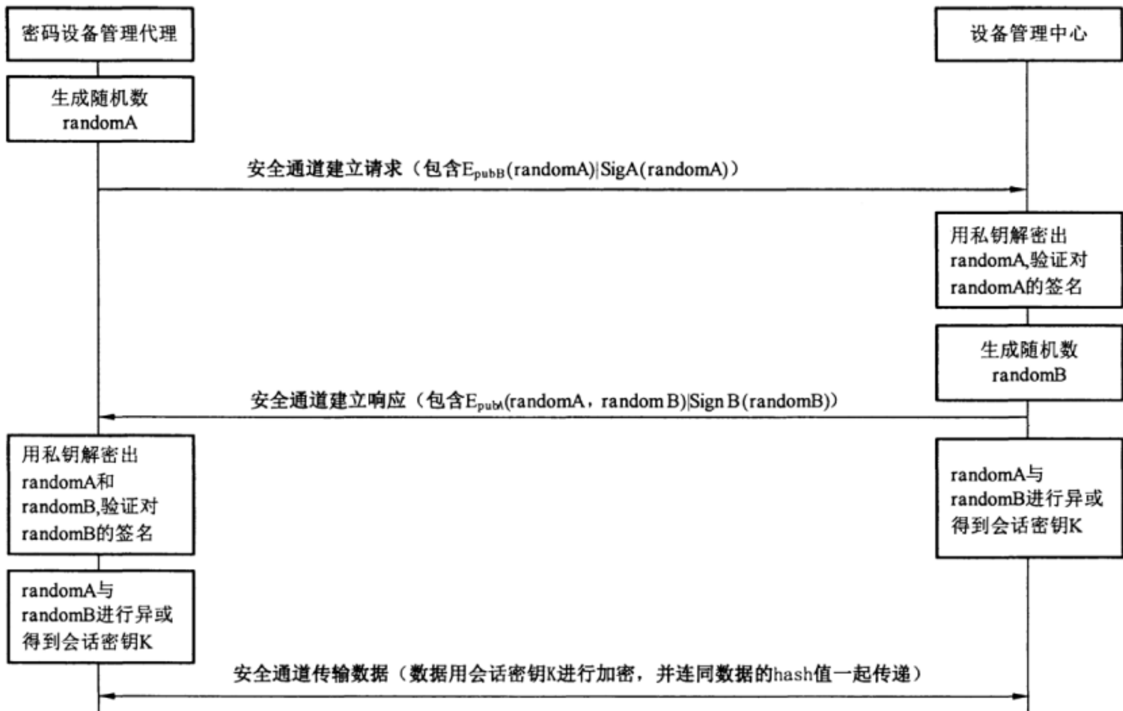
图 B.1 设备安全通道协议流程图
