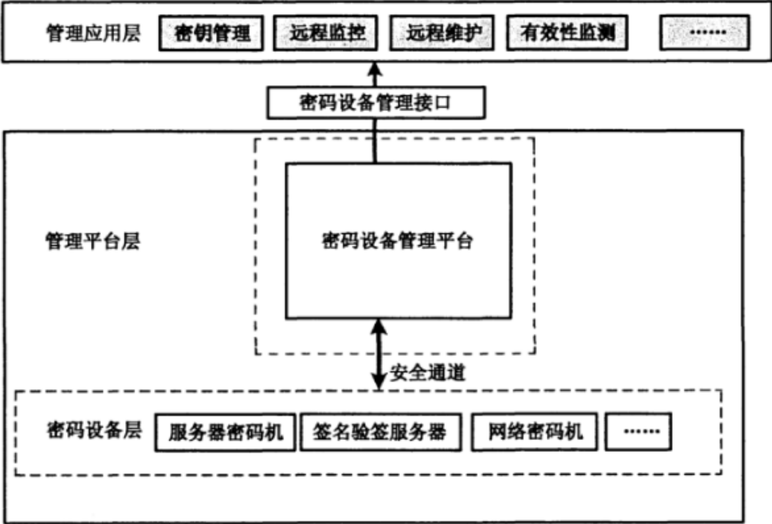
图 2 密码设备管理应用体系结构图
