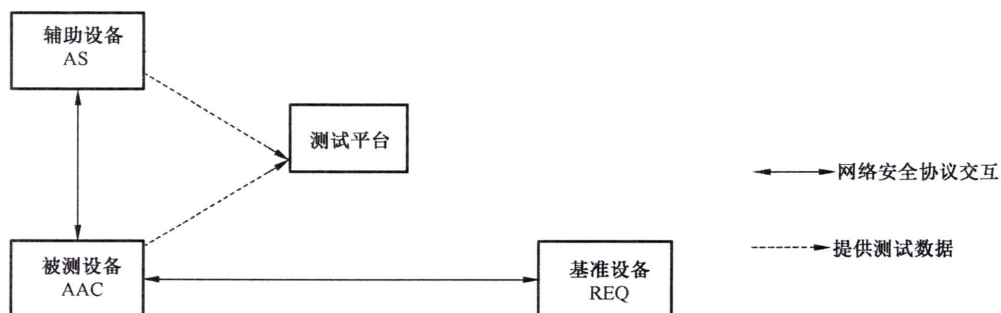
图 2 AAC 测试拓扑
