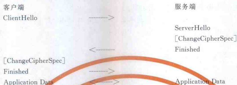
图 2 重用的握手消息流程
