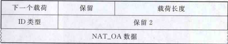
图 16 NAT_OA 载荷格式
