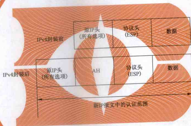
图 28 IPv4 的 AH 传输模式
