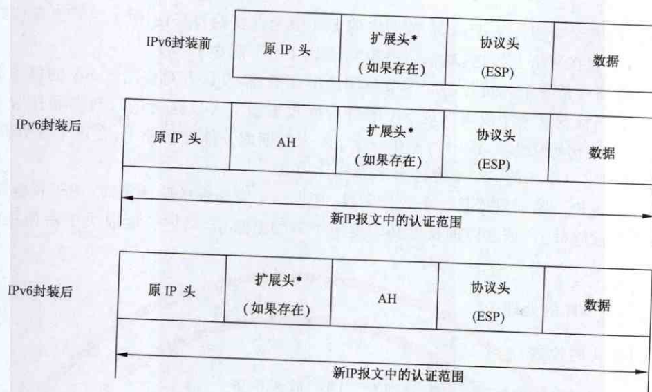
图 29 IPv6 的 AH 传输模式
