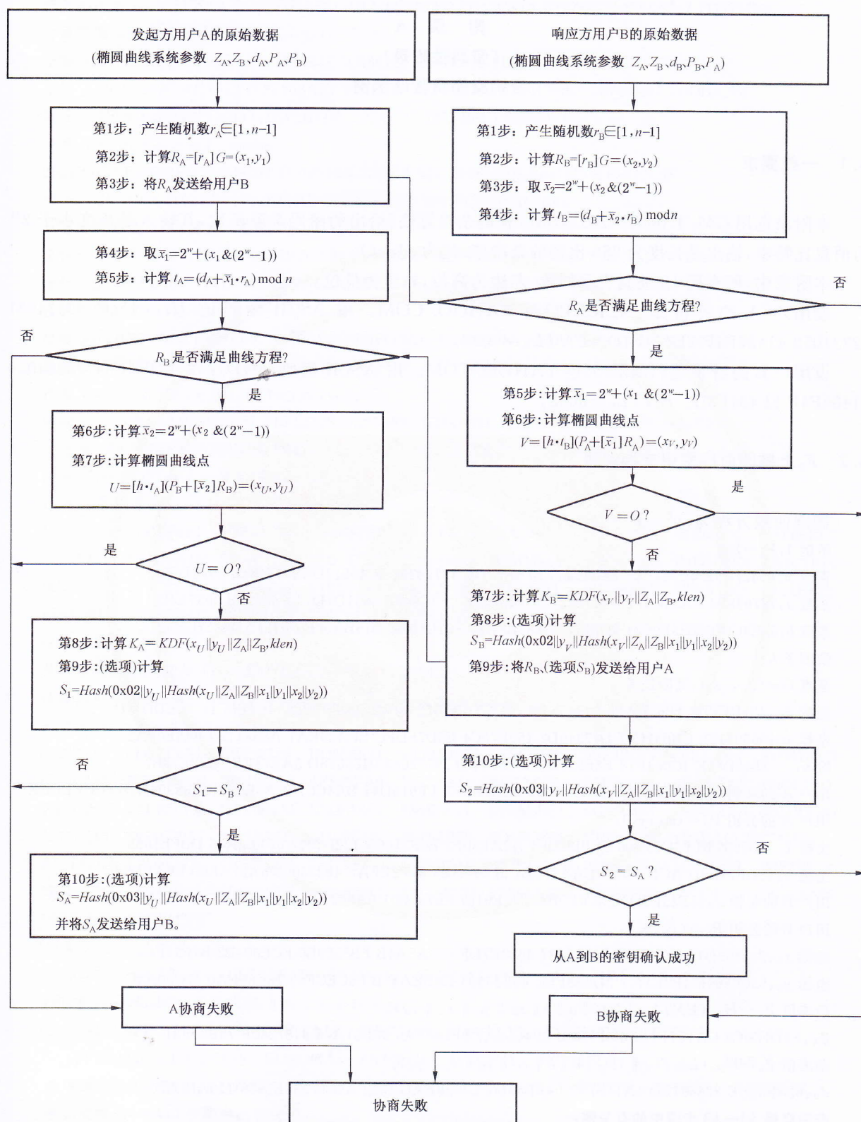
图 1 密钥交换协议流程
